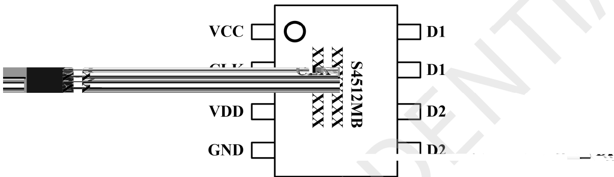
图 3 封装管脚图
